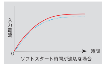
— 試験する機器の立上がり時間 - - - 本製品の立上がり時間
